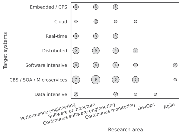
Fig. 21. Methodologies/techniques - Simulation.
